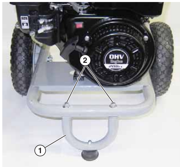
Figura 21 – Instalación del soporte delantero
