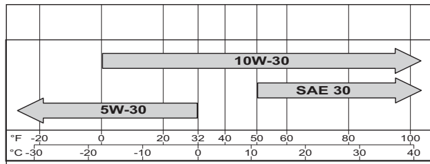
Figura 52 – Aceite recomendado
