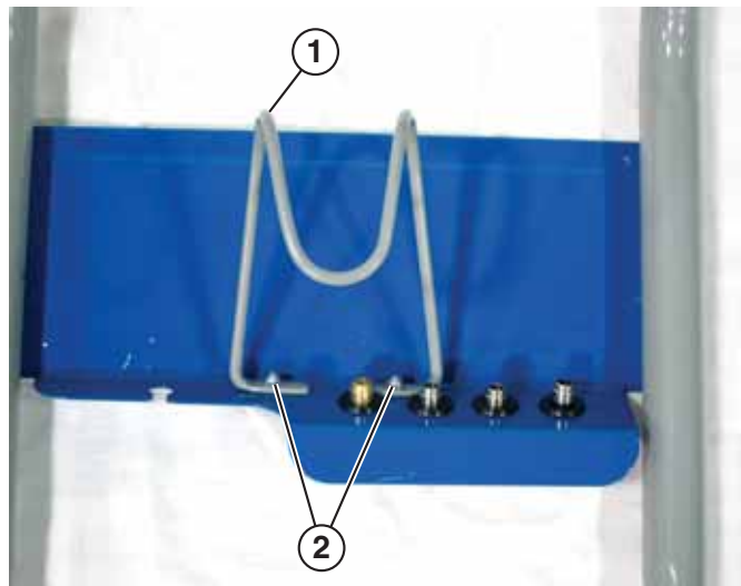
Figura 11 – Instalación del soporte de la manguera
