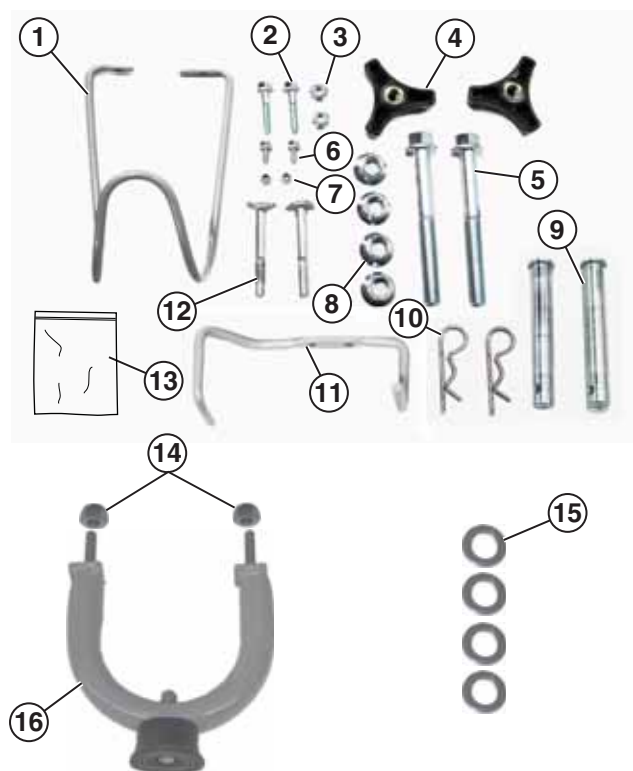
Figura 5 – Hardware
