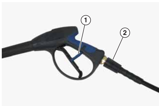
Figura 26 – Bloqueo del disparador en posición OFF (apagado)
