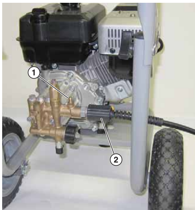
Figura 25 – Instalación de la manguera de alta presión – WP3000Z
