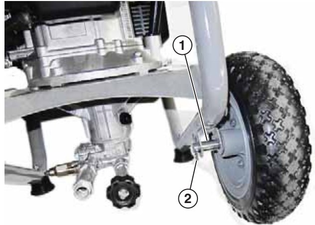
Figura 10 – Instalación del eje de la rueda
