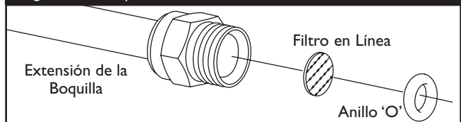
Figura 42 - Limpieza del Filtro
