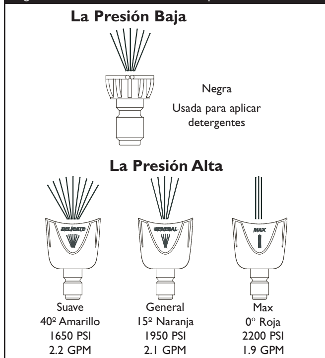
Figura 36 — Rocíe los Modelos del Boquilla
