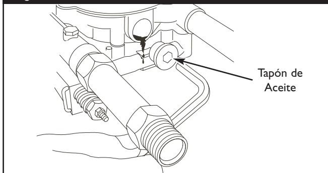
Figura 45 - Cambio del Aceite de la Bomba
