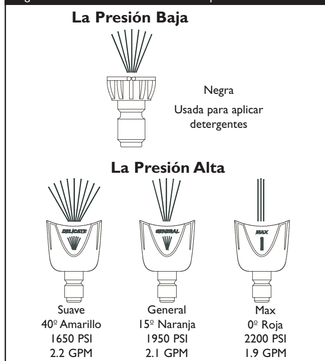
Figura 38 — Rocíe los Modelos del Boquilla
