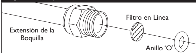
Figura 44 - Limpieza del Filtro
