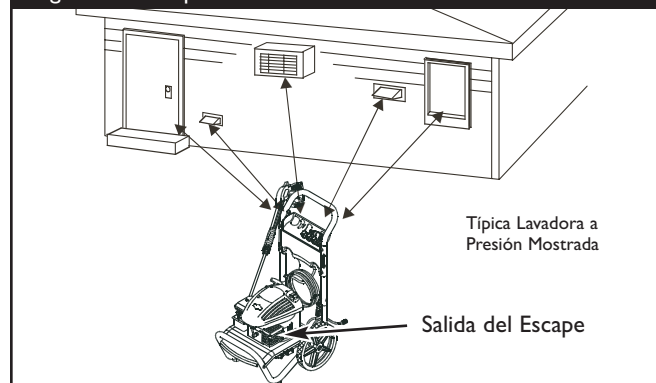
Figura 24 — Espacio Libre Alrededor del Lavadora a Presión
