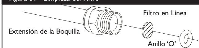
Figura 31 - Limpieza del Filtro
