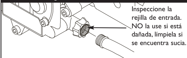
Figura 23 - Conecte la Manguera para el Jardín, a la Entrada de Agua
