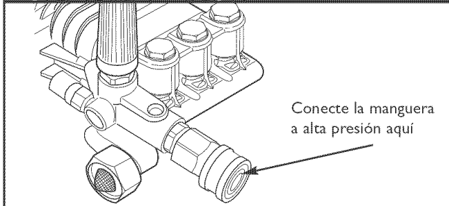
Figura 20 — Conecte la Manguera a Alta Presión, a la Bomba
