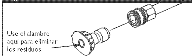
Figura 28 - Mantenimiento de la Extensión para Boquilla
