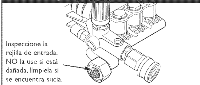
Figura 21 - Conecte la Manguera para el Jardín, a la Entrada de Agua
