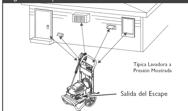
Figura 22 — Espacio Libre Alrededor del Lavadora a Presión
