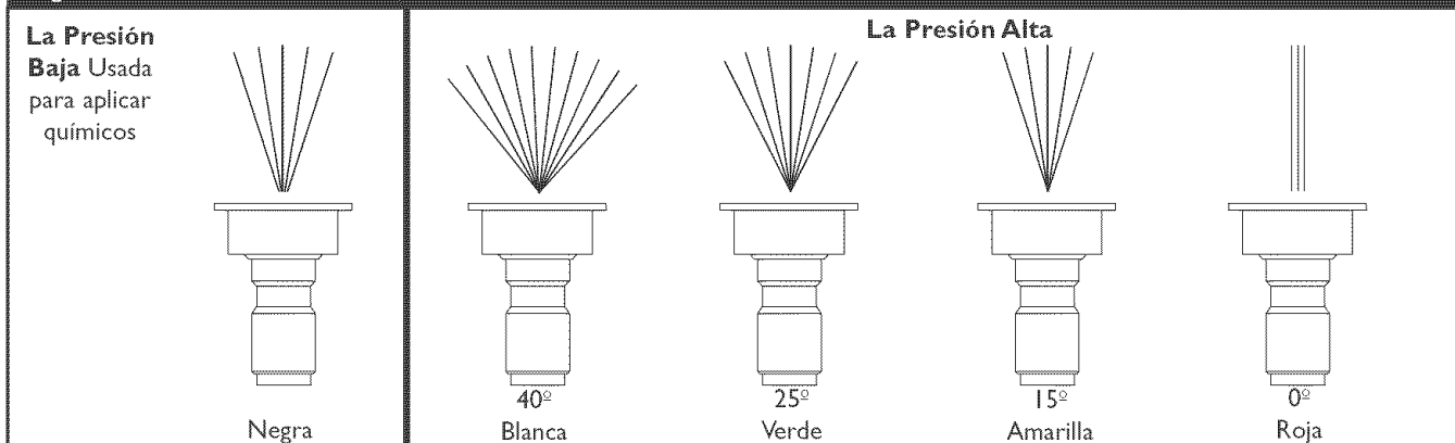
Figura 26 - Punta de Rociado
