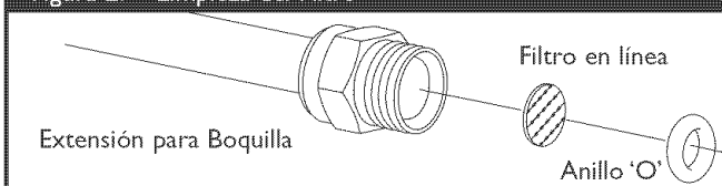
Figura 27 - Limpieza del Filtro
