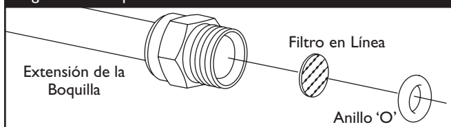
Figura 46 - Limpieza del Filtro
