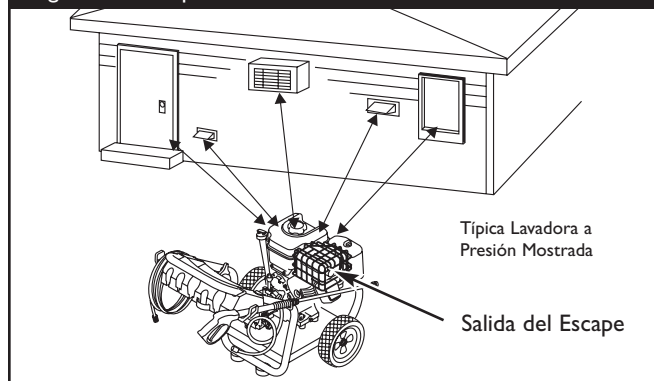
Figura 21 — Espacio Libre Alrededor del Lavadora a Presión
