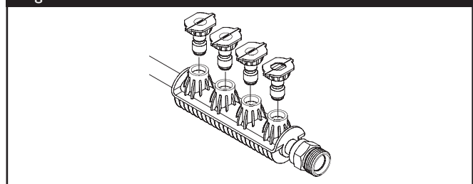
Figura 25 - Instale Puntas de Rocío en el Poseedor
