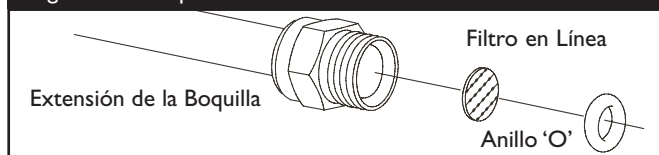
Figura 30 - Limpieza del Filtro
