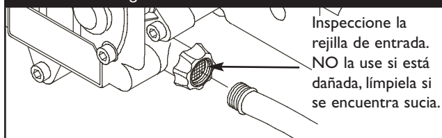
Figura 22 - Conecte la Manguera para el Jardín, a la Entrada de Agua
