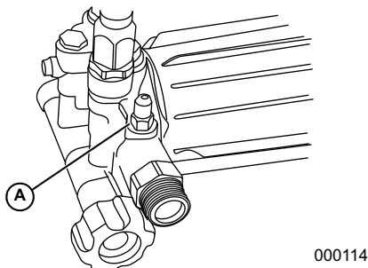
Figura 2-4. Conexión del tubo de sifón
