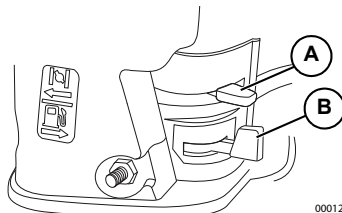
Figura 3-2. Válvula de combustible y cebador
