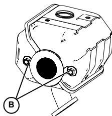
Figure 4-10. Fixations du pare-étincelles
