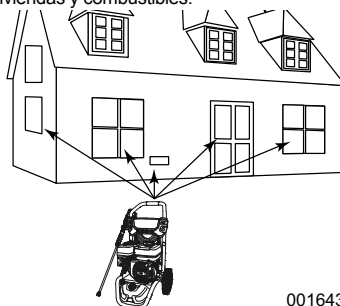
Figura 3-1. Cinco pies (1.5 m) de separación mínima
