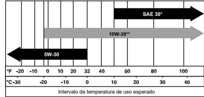
Figura 4-4. Viscosidad del aceite
