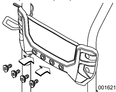
Figura 2-3. Inserción de las boquillas
