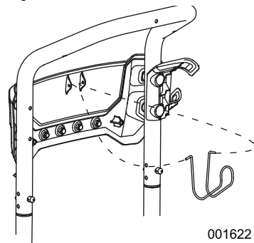
Figura 2-2. Instalación del gancho para manguera
