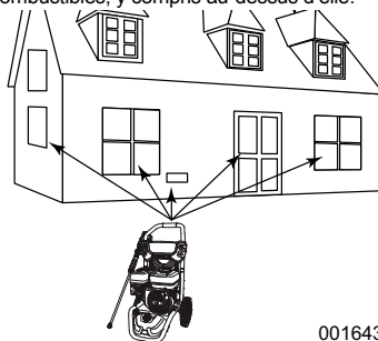
Figure 3-1. Dégagement d'au moins cinq pieds
