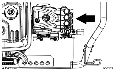
Figure 3-12. Déplacement de la pompe vers le moteur
