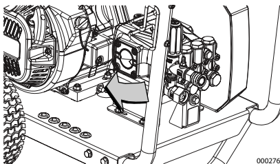
Figura 3-17. Tapón de vaciado de aceite
