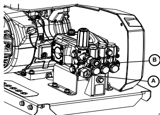
Figure 2-9. Raccord de l'alimentation en eau
