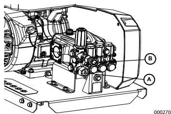
Figura 2-9. Conexión del suministro de agua
