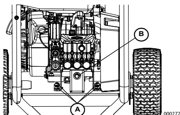
Figure 3-11. Desserrage des écrous
