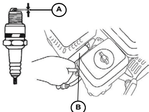
Figura 3-19. Bujía
