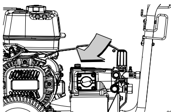
Figure 2-6. Vérification du niveau d'huile de la pompe
