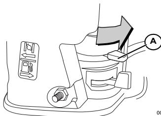
Figura 3-5. Válvula de combustible y cebador
