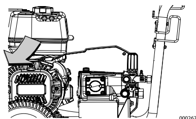
Figura 2-6. Comprobación del aceite de la bomba
