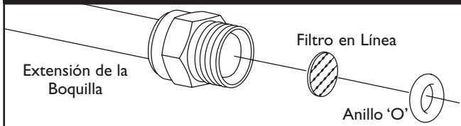
Figura 29 - Limpieza del Filtro
