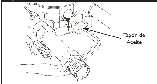
Figura 32 - Cambio del Aceite de la Bomba
