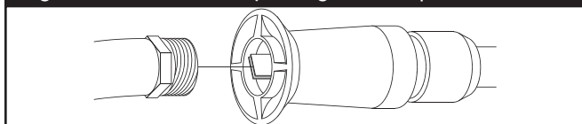
Figura 31 - Suministrar Flujo de Agua a la Boquilla
