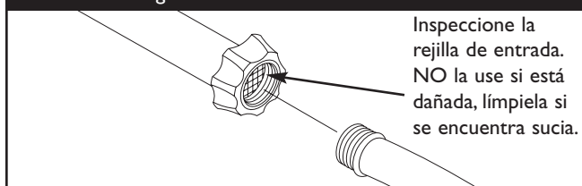
Figura 22 — Conectar la Manguera del Jardín a la Entrada de Agua
