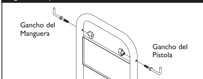
Figura 19 - Fijar el "L" Perno a la Manubrio
