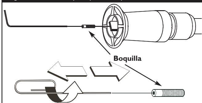
Figura 30 - Remover y Limpiar la Boquilla
