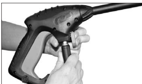
Figura 3 - Conecte la manguera de alta presión a la pistola (todos los modelos)
