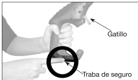
Figura 8 - Pasador de seguridad del gatillo
