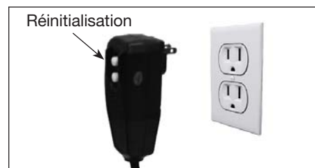
Figure 9 - Prise de terre/bouton de réinitialisation
