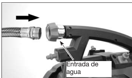
Figura 7 -Conecte la manguera de jardín a la unidad
