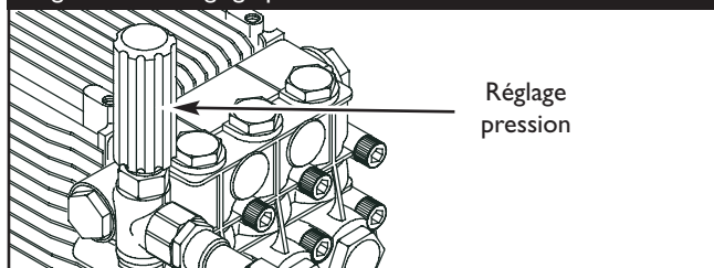
Figure 35 — Réglage pression
