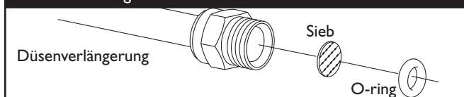
Abb. 56 - Reinigen des internen Siebs
