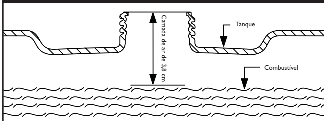
Figura 66 — Espaço de Expansão de Combustível Típico
