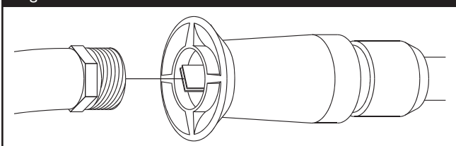
Figure 31 — Rincez Pendant le Gicleur
