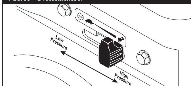
Abb. 53 - Drosselsiebel
