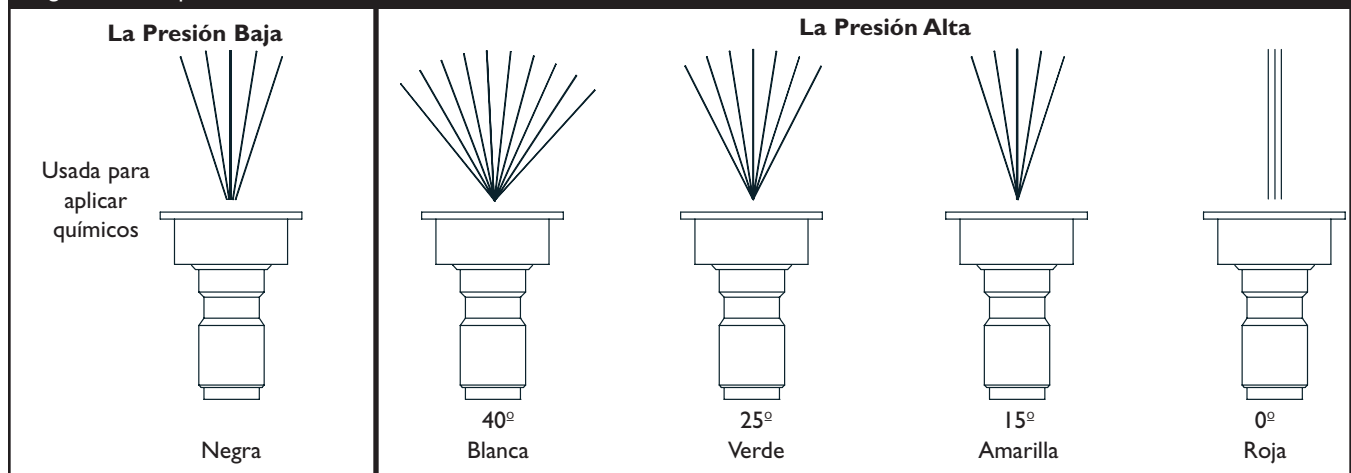
Figura 24 - Boquillas
