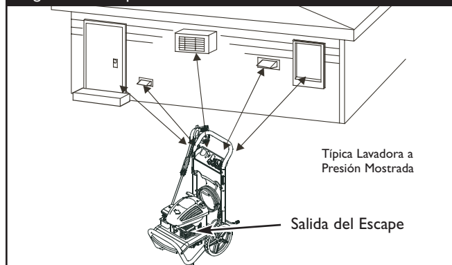
Figura 32 — Espacio Libre Alrededor del Lavadora a Presión
