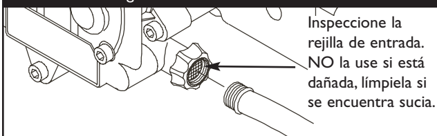
Figura 31 - Conecte la Manguera para el Jardín, a la Entrada de Agua
