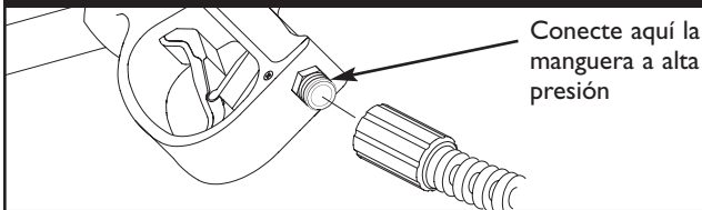
Figura 29 - Conecte la Manguera a Alta Presión a la Pistola Rociadora
