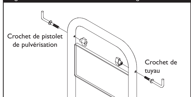
Figure 17 - Fixez les Crochets en "L" à la Poignée
